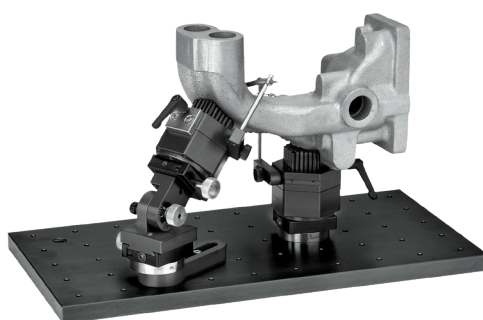
SWA39-System und NADELFIX auf SPANNFIX ECO Baseplate
