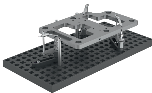
Einsatz des Start-Kits auf einer QUADERFIX -Platte
